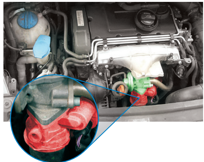
Blick in den Motorraum eines VW Tourans grün hervorgehoben: AGR-Ventil; rot hervorgehoben: Regelklappe
